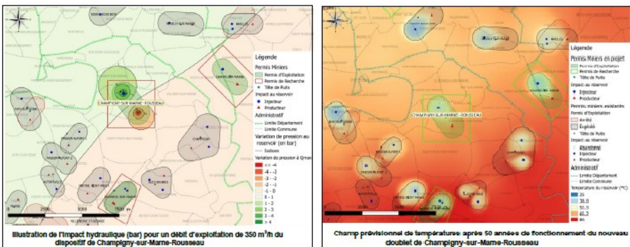
Illustration 13: cartographie des impacts hydrauliques de l'exploitation de la nappe par le doublet "Rousseau" Source : dossier (pp. 104 et 106)
