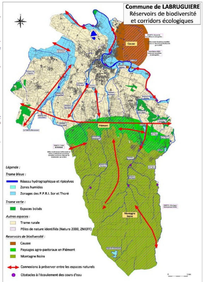
Figure 26 : Eléments de la trame verte et bleue
