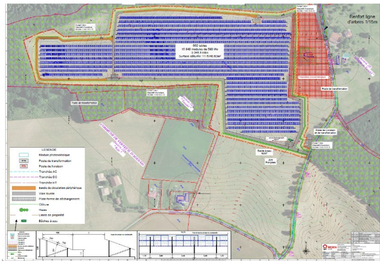
Figure 6 : Plan masse du projet de parc photovoltaïque - source : REDEN
