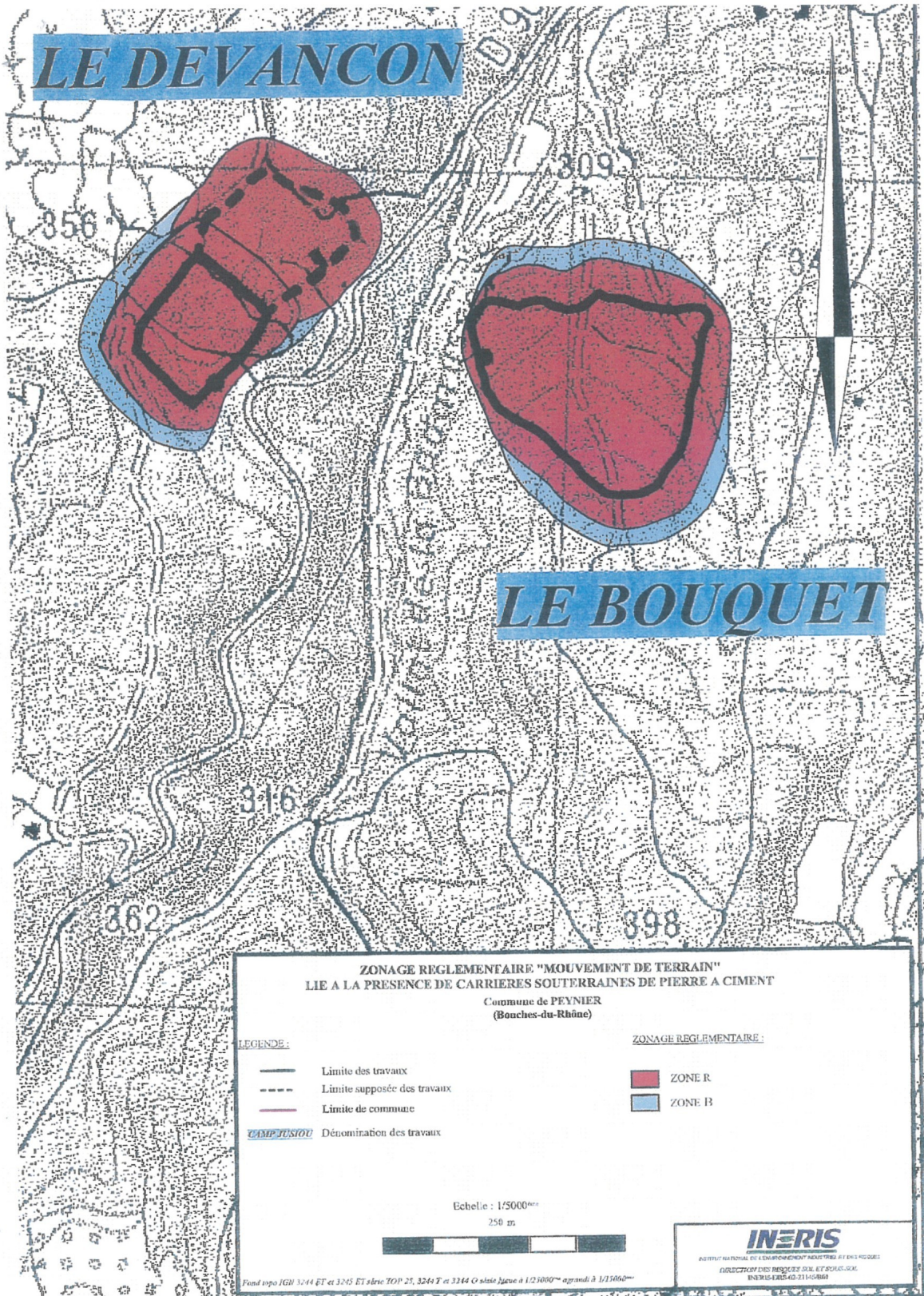
Illustration 2: Carte de zonage du PPR Carrières souterraines de pierre à ciment existant (approbation 2009)
