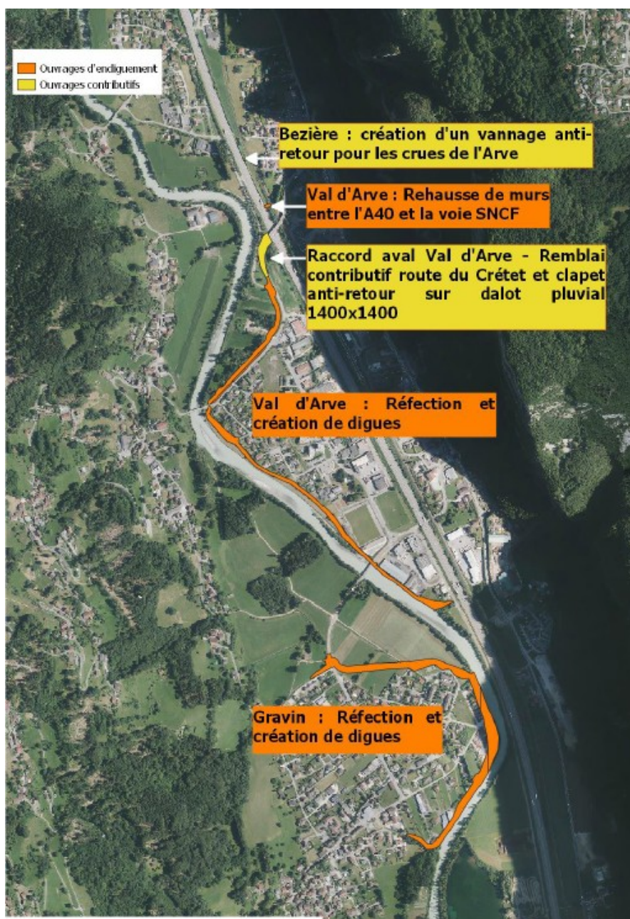
Illustration 2 : Système d'endiguement projeté. Source : étude de danger.
