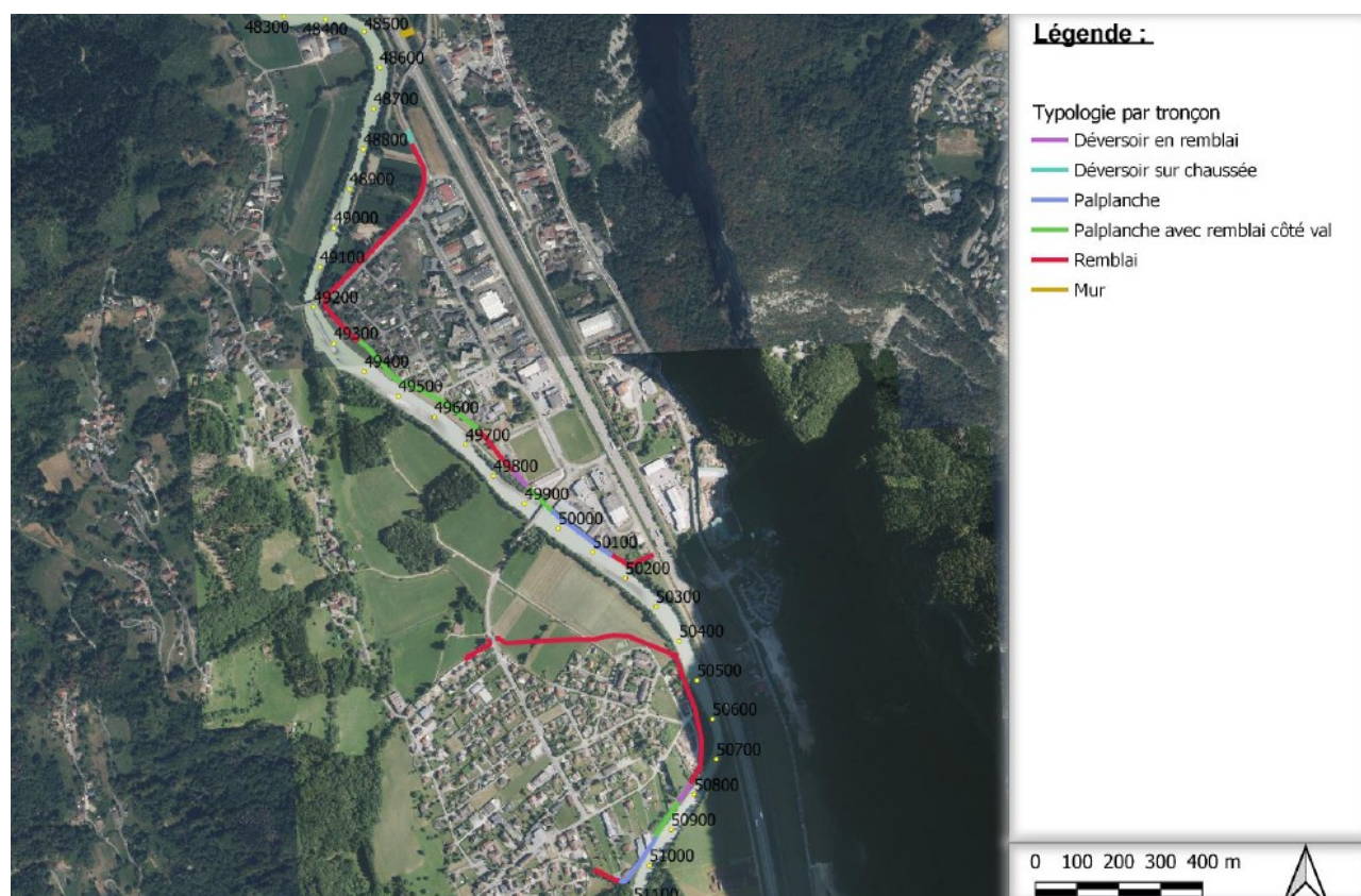
Illustration 1 : Localisation des principaux ouvrages du système d'endiguement de Magland. Source : étude de danger
