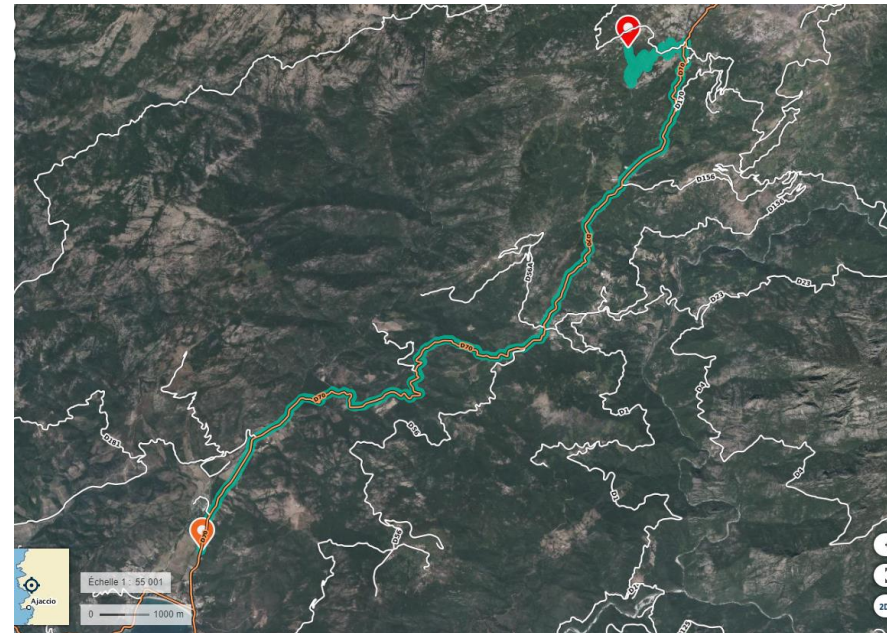
Figure 3 : Tracé prévisionnel du raccordement externe de la centrale photovoltaïque
