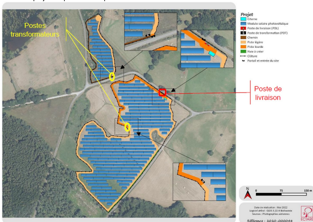
Plan masse du projet – extrait étude d'impact page 22
