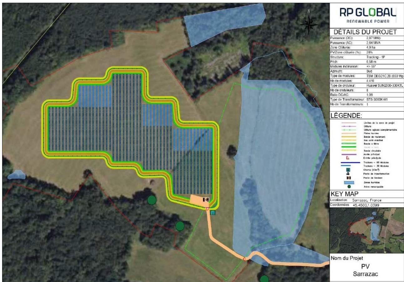
Plan masse projet - extrait étude d'impact page 38
