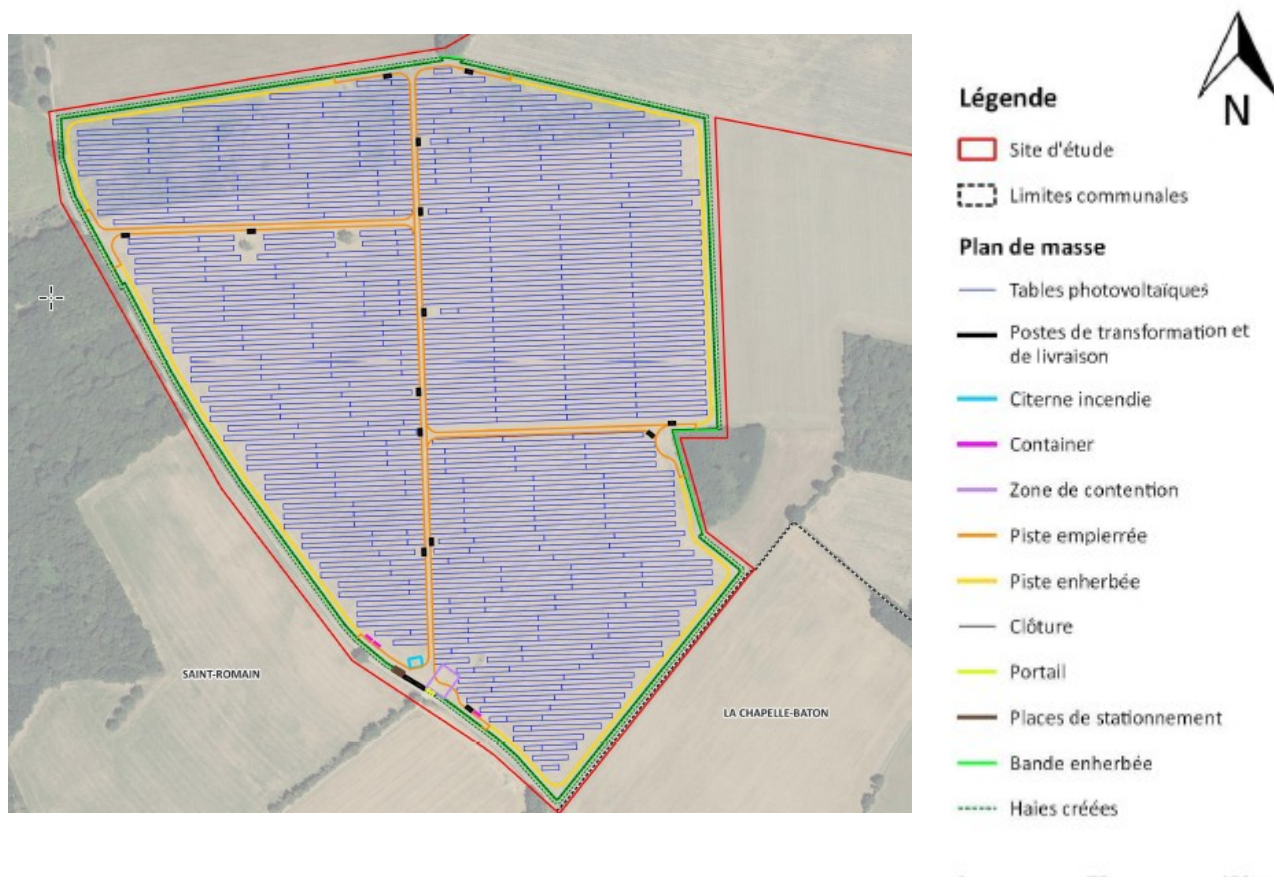
Plan masse – extrait étude d'impact page 65
